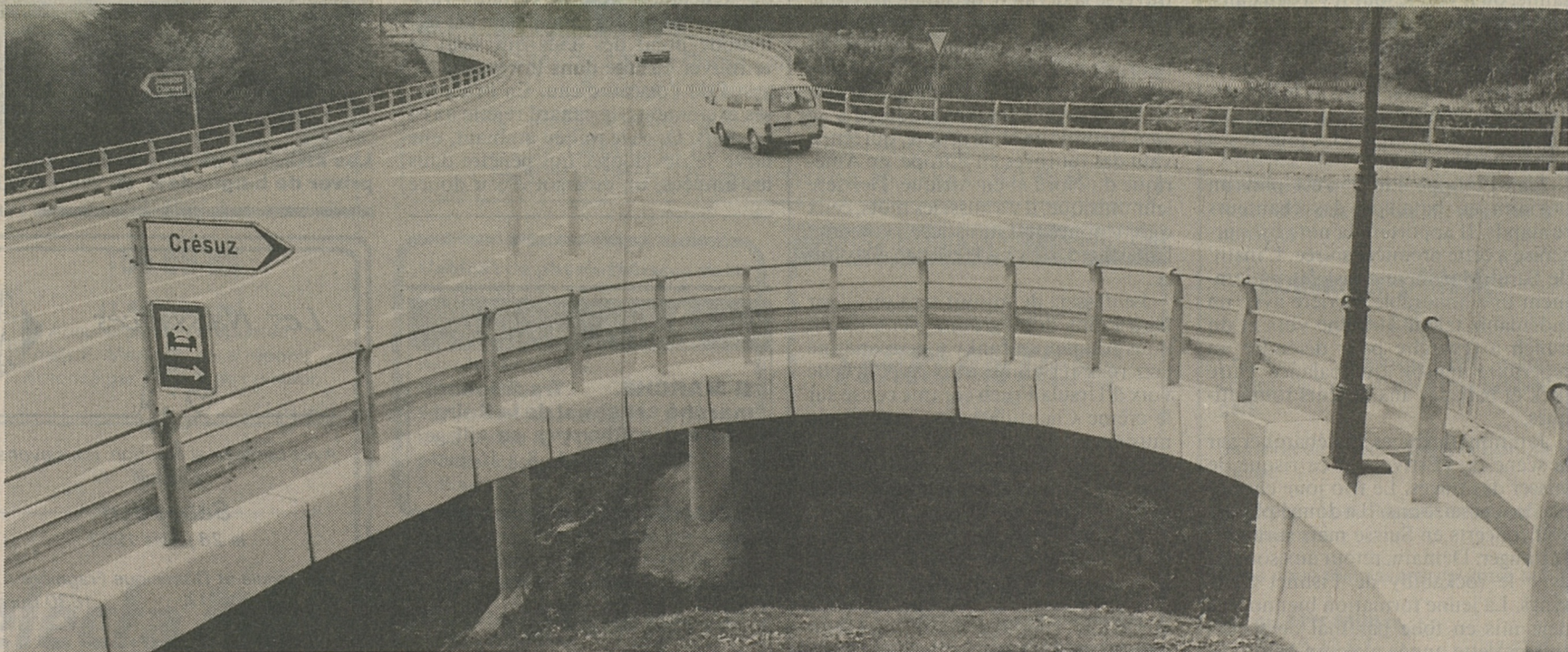
En haut, le pont sur la Sarine, premier de ce type à avoir une portée supérieure à 100 mètres, et le pont sur la Glâne, premier pont courbe lancé de Suisse. Jean Mülhauser En bas, le pont de la Maladeire, à Crésuz, fort complexe sur le plan des calculs et de la réalisation. Mayard-a
