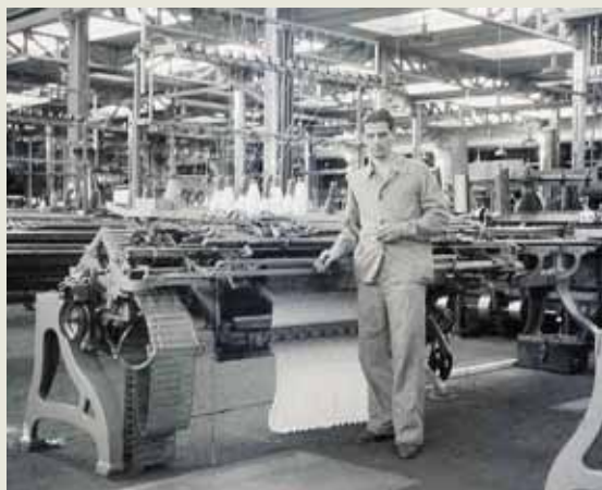
Machine à tricoter Dubied. AVEC L'AIMABLE AUTORISATION DE MICHEL JEANNERET, PHOTO PERSONNELLE PUBLIÉE SUR LE SITE HTTP://WWW.NOTREHISTOIRE.CH/
