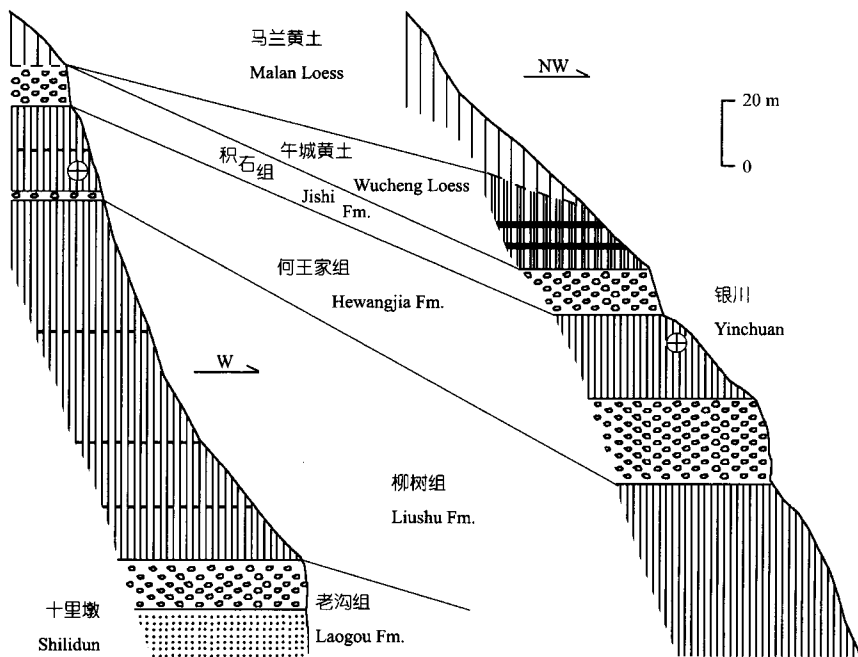
图7 十里墩和银川地点剖面图(图例见图2)
