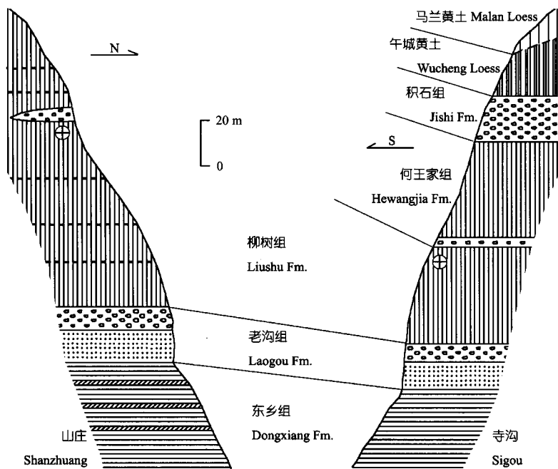
图8 山庄和寺沟地点剖面图(图例见图2)
