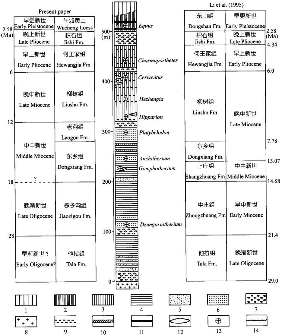
图2 临夏盆地新生代地层综合柱状图
