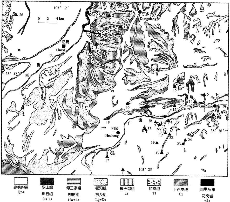
图 1 临夏盆地哺乳动物化石地点分布
