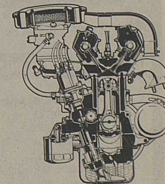
Le moteur de la 131 Racing n'est pas un inconnu non plus. Ce 2 litres équipait déjà, notamment, le fameux coupé 124 Sport. On le reconnaît en particulier à son double arbre à cames en tête. Sa puissance: 115 ch DIN.
