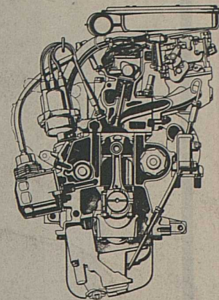
Mécanique éprouvée, pour la 127 Sport, puisqu'il s'agit du 1049 cm 3 à arbre à cames en tête. Après quelques « retouches », il développe 70 ch DIN.
