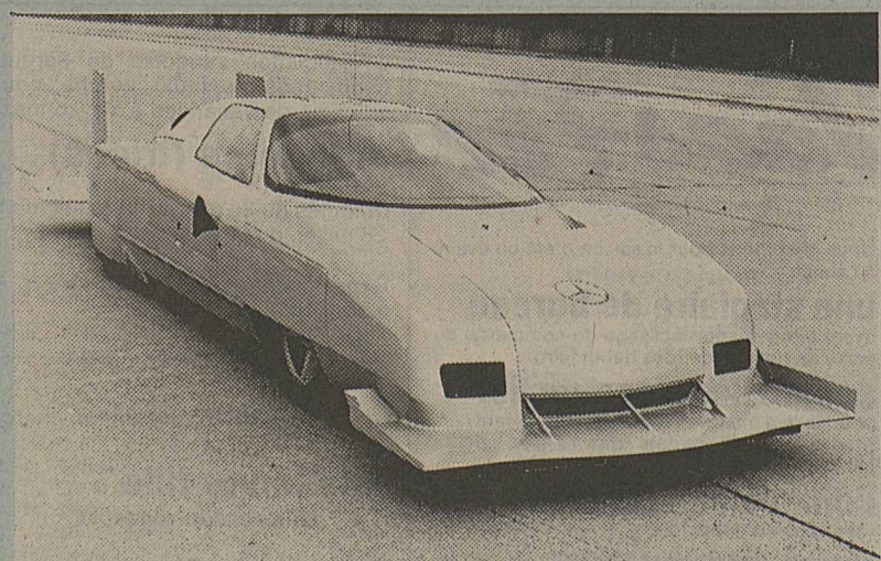
Plus de 400 km/h.: la Mercedes C 111/IV qui établit cinq nouveaux records du monde absolus sur le circuit de Nardò, franchissant notamment la barrière des 400 km/h. pour la première fois sur un tour avec 403,978 km/h. La C 111/IV est équipée d'un moteur à essence V8 turbo-compressé de 500 ch.
