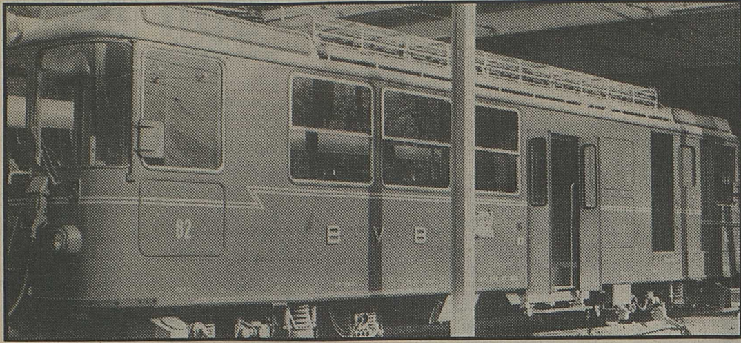
La dernière automotrice datant d'il y a deux ans et que l'on désigne par la « 82 ».
