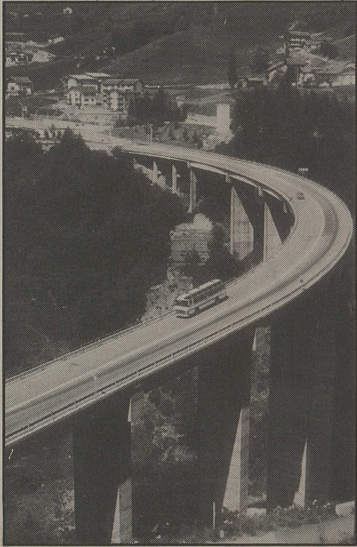
Autres temps, autres moyens. Ici, le fameux viaduc de Bosses avec ses 72 m de haut, une des pièces maîtresses de la nouvelle route du Grand-Saint-Bernard.
