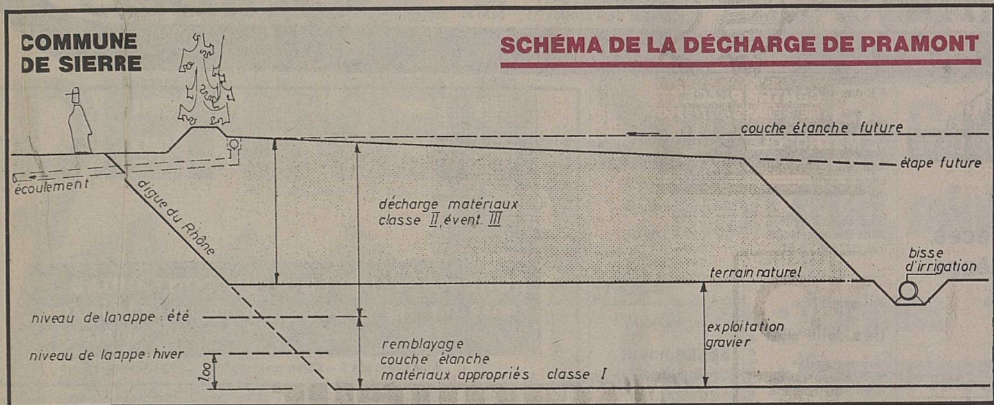
Le schéma d'une décharge, ici celle de Pramont: des normes rigoureuses.
