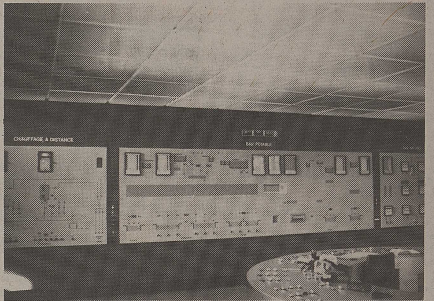
Une vue du tableau de commande automatique du réseau d'eau pour le gaz et l'électricité.
