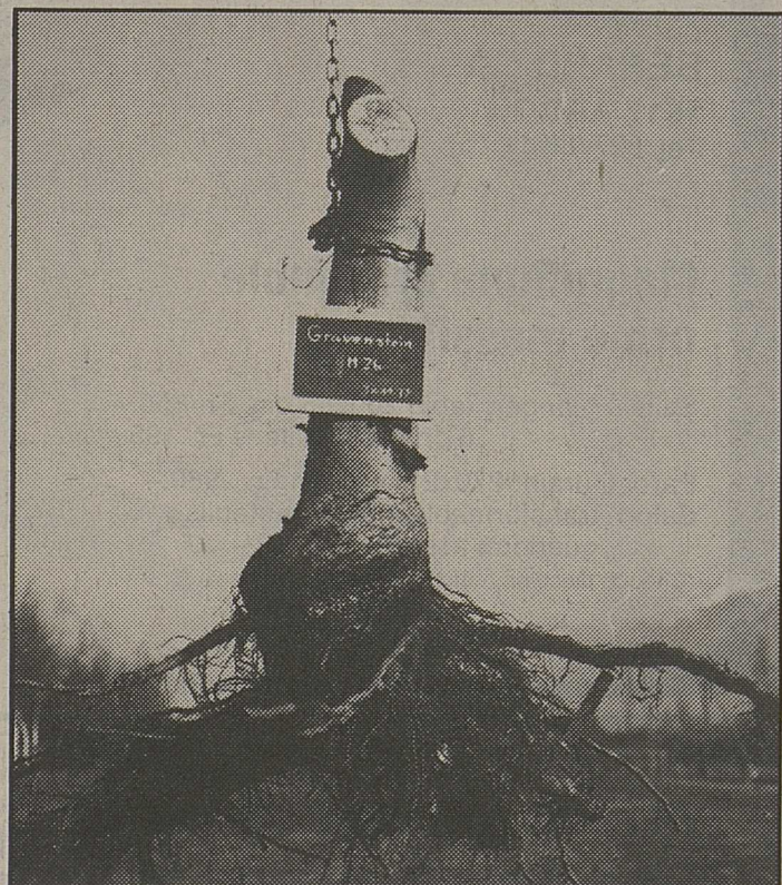
Un exemple de porte-greffe expérimenté sur un gravenstein
