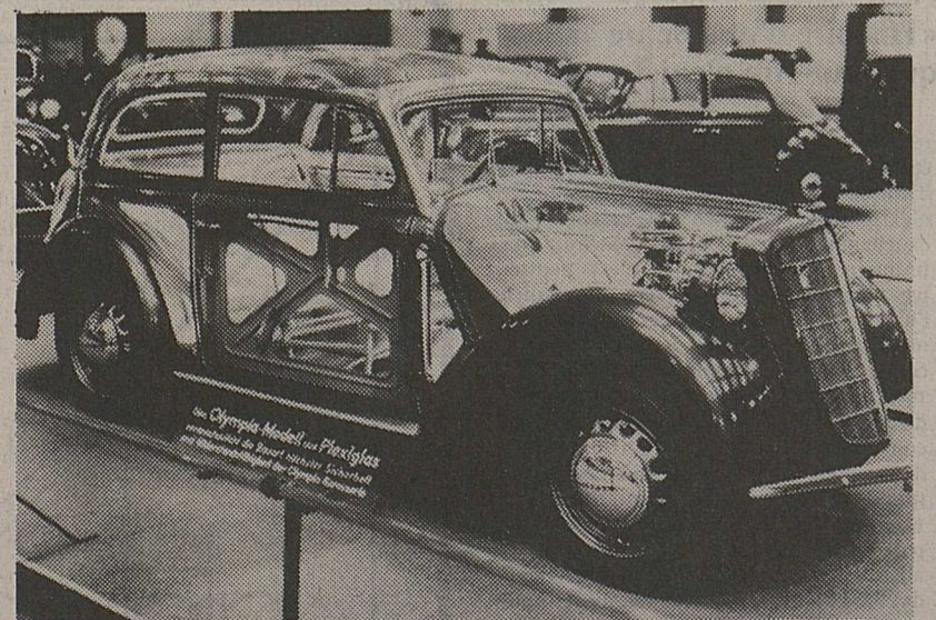
Une coupe de l'Opel Olympia, exposée au Salon de Berlin en 1937. C'était la première voiture de série européenne dont le moteur et les essieux n'étaient plus montés sur un cadre mais fixés directement à la carrosserie « autoporteuse ». Des patentes Opel protègent la construction (DRD 745079) et le montage (DRP 765899). A l'encontre de ce que pensaient les gens de l'époque (soit que la carrosserie autoporteuse pourrait se briser en route), l'Olympia s'est avérée une voiture extrêmement robuste et sûre. Dans l'intervalle, cette conception lancée il y a 40 ans par Opel s'est imposée dans le monde entier. C'est en effet sur ce procédé que repose la conception de l'habitacle formant cellule de sécurité et entouré de zones de déformation.
