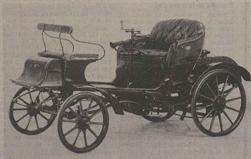
Automobile Opel 4 ch « Système Lutzmann »; année de construction 1898; vitesse 18-20 km ; prix : avec pneus pleins 4000 marks, avec pneus gonflables 4300 marks. Moteur arrière, refroidissement à eau ; huilage à la burette ; soupapes automatiques ; entraînement par chaîne sur les roues arrière ; deux vitesses et marche arrière ; changement de vitesse sous le volant.
