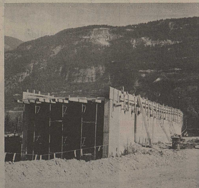
Dernier ouvrage actuellement en construction avant le viaduc de Riddes : ce tunnel en béton armé est destiné à conduire, par le canal de fuite, les eaux turbinées à la centrale électrique FMM d'Ecône, jusqu'au Rhône.
