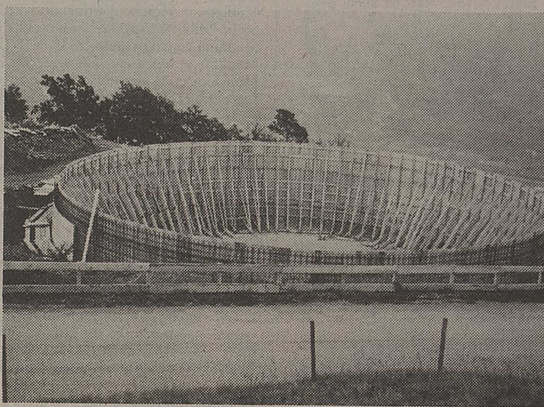
L'imposant coffrage du réservoir circulaire, actuellement en construction.
