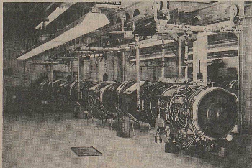
Des réacteurs du «Tiger» au banc d'essai dans les ateliers Northrop à Palmdale.
