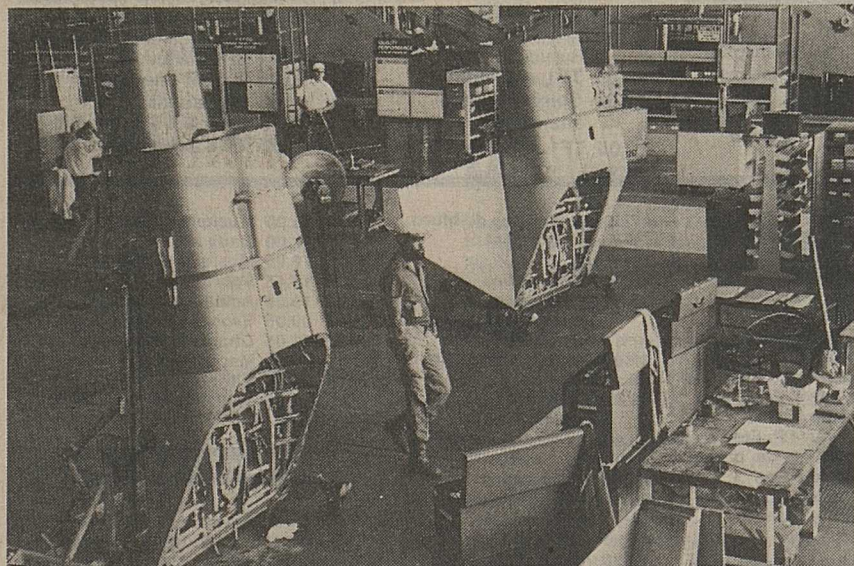
Des parties arrières du «Tiger» dans les ateliers de montage Northrop à Hawthorne près de Los Angeles.
