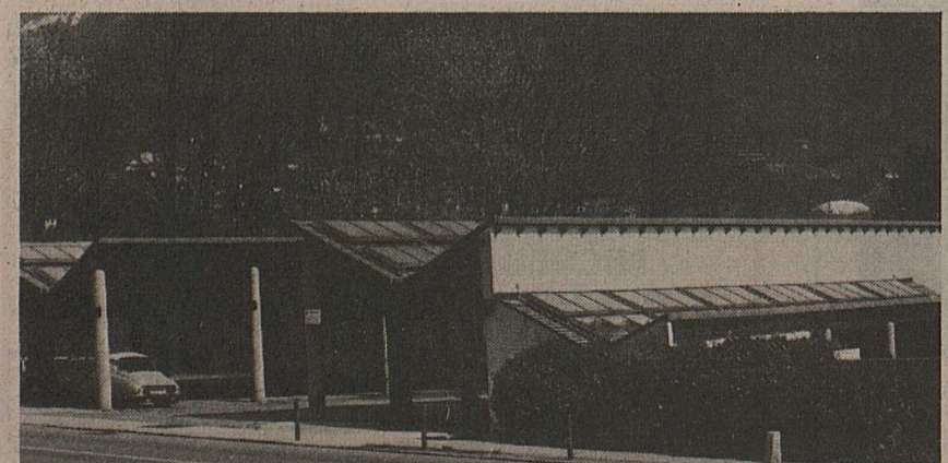
Depuis la mi-juillet 1977, l'eau sanitaire et celle de la piscine du village de vacances M (140 personnes) à Lugaggia (TI) est chauffée par l'énergie solaire. L'économie annuelle de mazout dépassera les dix tonnes, ce qui représente une réduction d'au moins 300 heures de chauffage.
