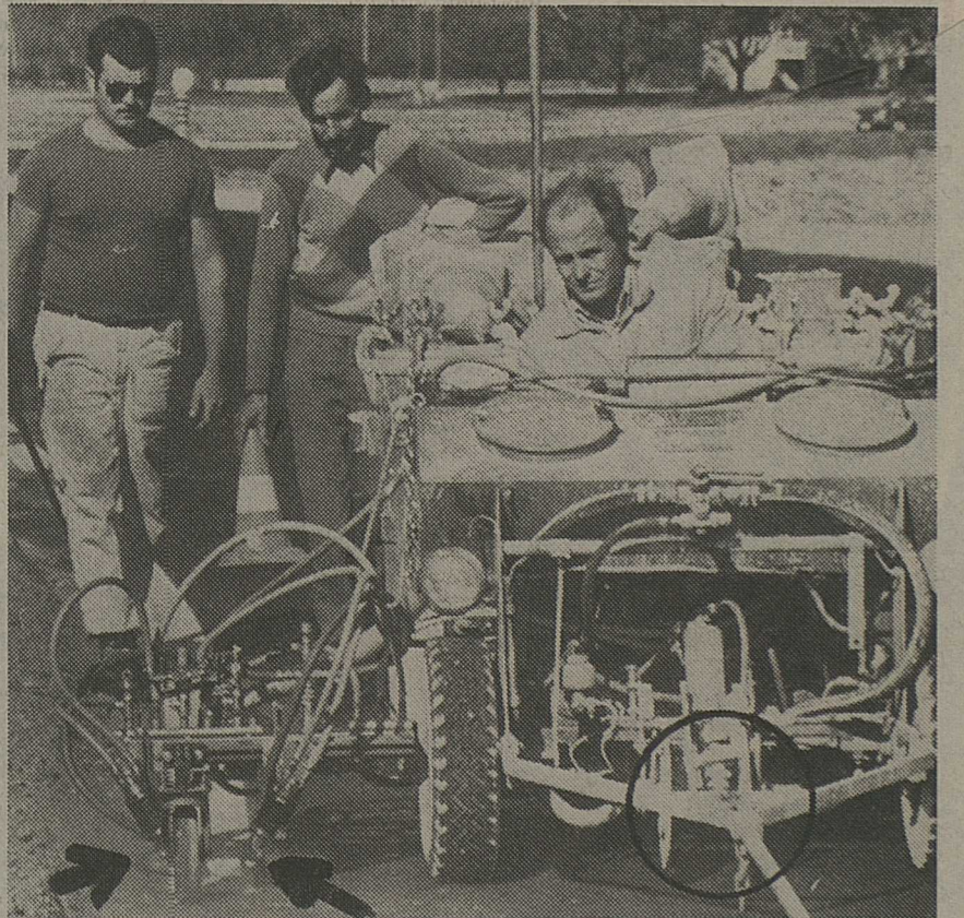
A gauche, les flèches indiquent la position des nouveaux gicleurs. On remarque la ligne blanche derrière les gicleurs. Au centre, dans le cercle, le double disque qui disparaîtra progressivement sur ces machines.
