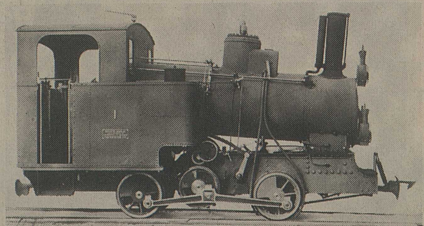
La locomotive à vapeur pour adhérence et crémaillère - une HG 2/2 - qui servit à la construction de la ligne du MC. Elle fut ensuite vendue à la Compagnie du tramway du Mont-Blanc, à Saint-Gervais.
