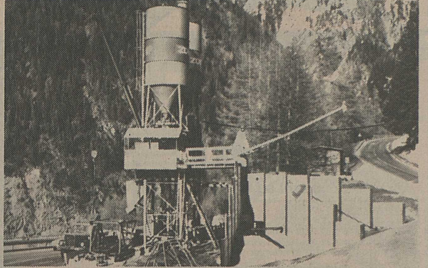
On installe sur place le matériel de fabrication du béton.
