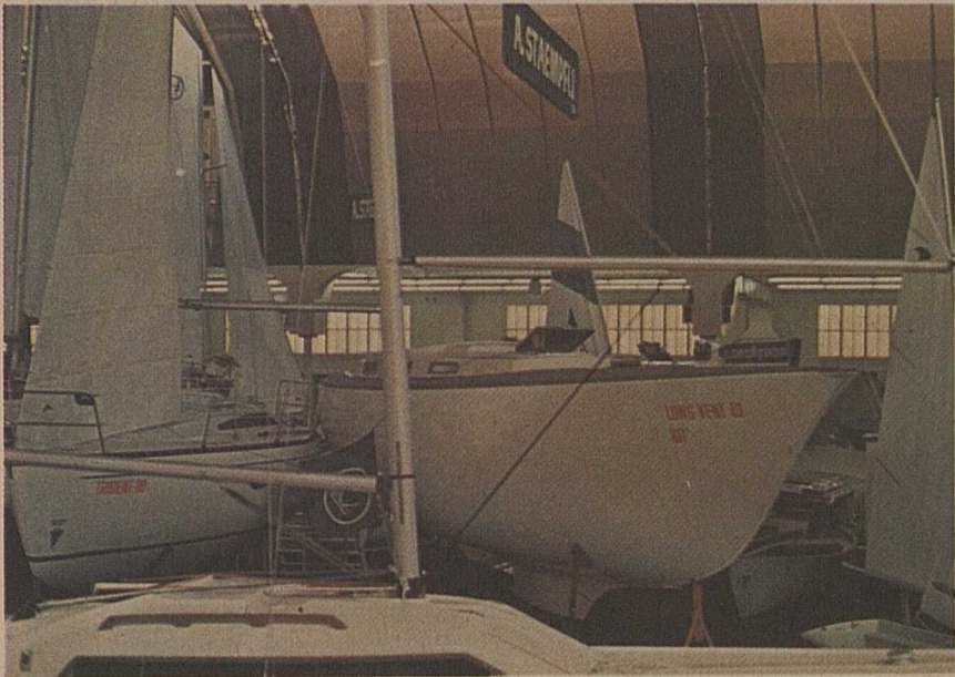
Un remarquable prototype de la maison Staempfli à Grandson : le voilier « Long-Vent » de 12 m de long. Première mondiale.
