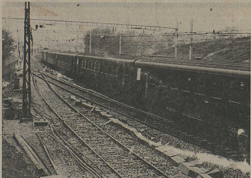
La courbe de l'entrée en gare de Nyon, côté Lausanne. Son rayon actuel exige un ralentissement à 115 km/h, sans compter une sensible perte de temps. Cet exercice revient annuellement aux CFF à quelque 130 000 francs, (consommation supplémentaire de courant, sabots de freins, notamment).
