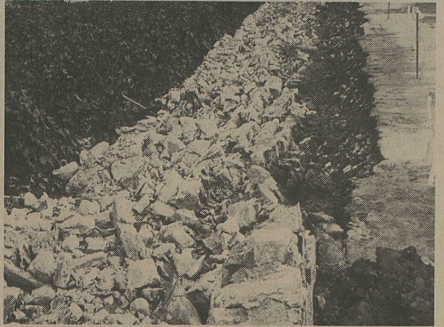
Le mur qui s'est couché dans la vigne.
