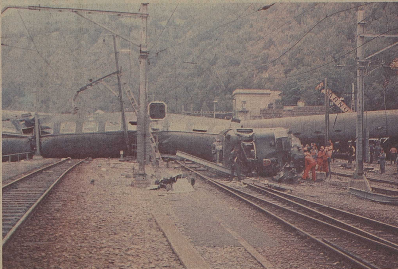
Une vue générale du déraillement. On remarque que les wagons se sont éparpillés dans les deux directions, la locomotive revenant pratiquement au centre des diverses voies.
