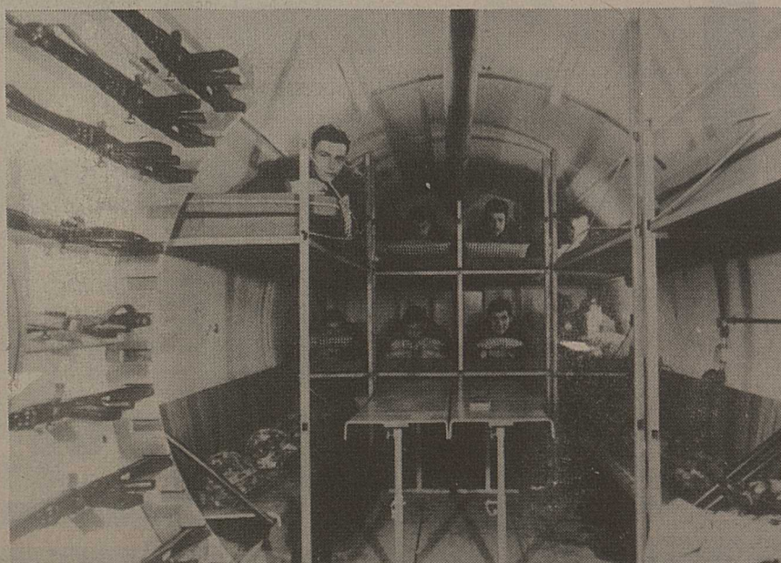
Les abris antiatomiques, dits AAA, jouent un rôle très important dans le domaine du renforcement du terrain. Leur but est de protéger les troupes qui mènent le combat défensif contre les actions directes et indirectes de l'ennemi et de leur permettre de survivre aux effets des armes de destruction de masse. Voici un local de travail et un abri aménagés dans un poste de commandement.
