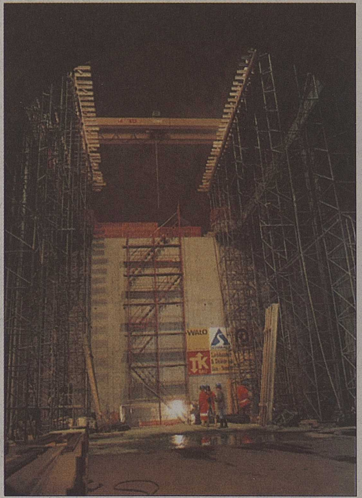
Deux concerts seront donnés par le festival dans l'énorme «caverne» de Bieudron.
