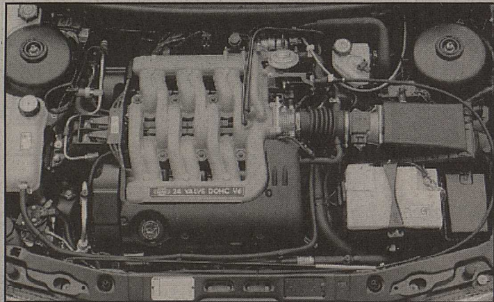
Le V6 très compact est installé transversalement. On remarque les doubles pipes d'admission, qui forment une jolie pièce de fonderie.
