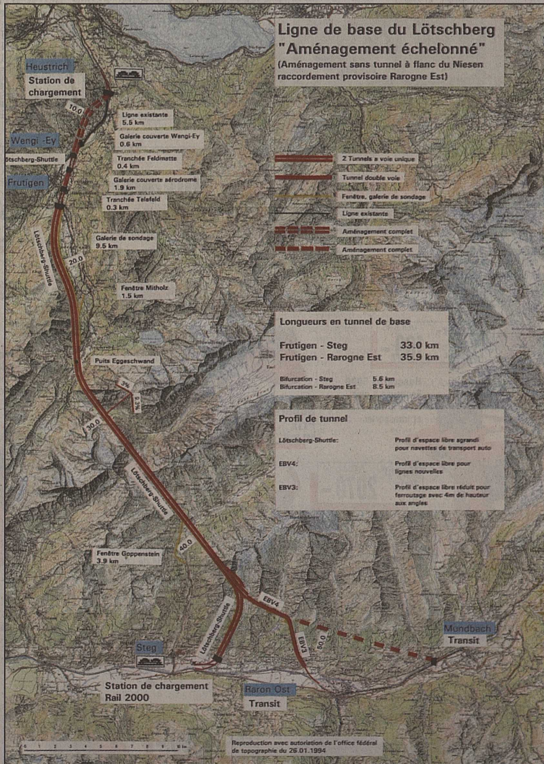
La variante par étapes à 4,22 milliards. Le Mundbach et le Niesen sont prévus dans une deuxième phase.
