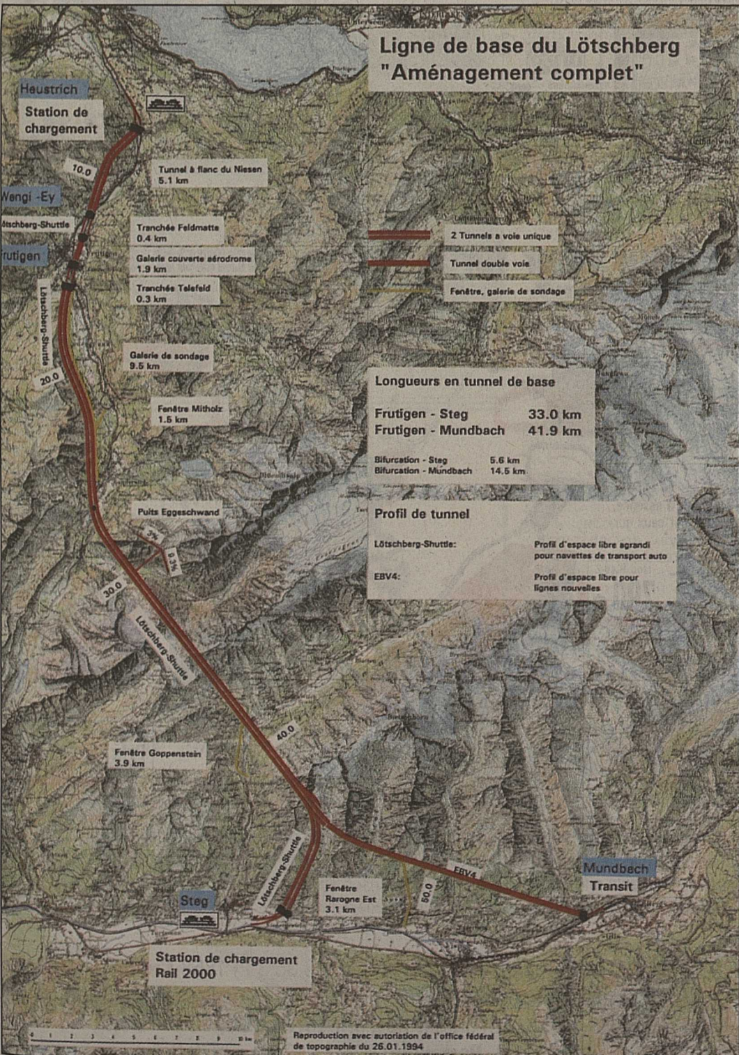
La variante complète à 4,93 milliards. Le prolongement jusqu'au Mundbach et le tunnel du Niesen seraient construits tout de suite.
