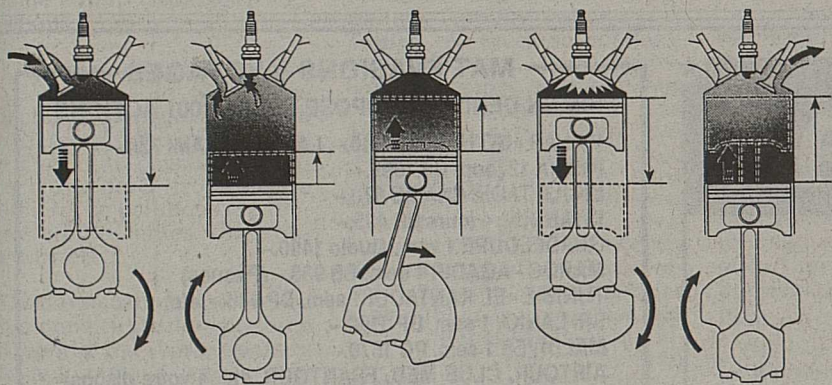
Admission Pas de compression Compression Expansion Echappement
