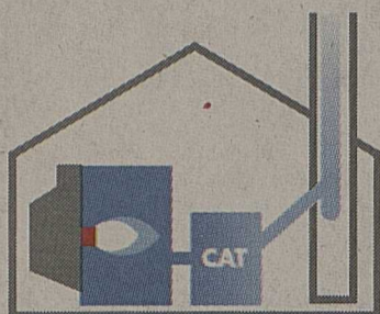
Chauffage au mazout moderne LOW-NO x à condensation et avec catalyseur pour installation d'une certaine importance.
