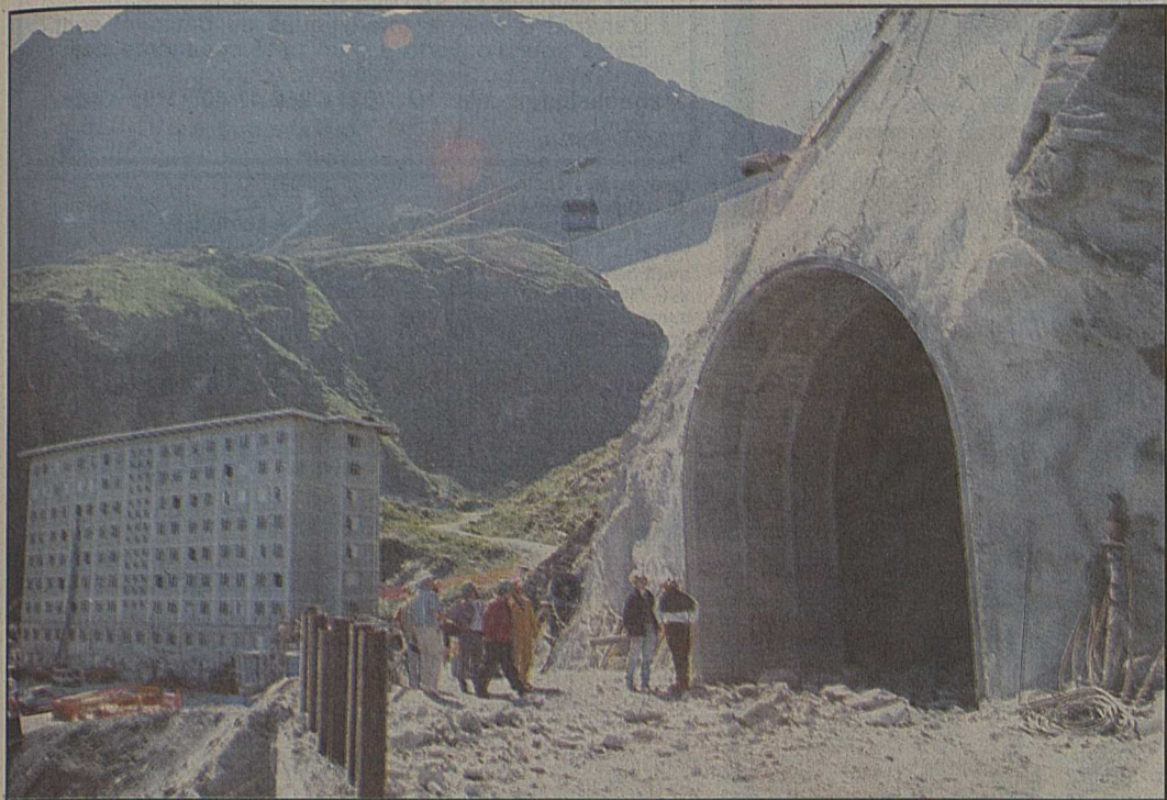
L'entrée de la galerie principale d'amenée d'eau qui a fait l'objet du «premier» coup de mine.
