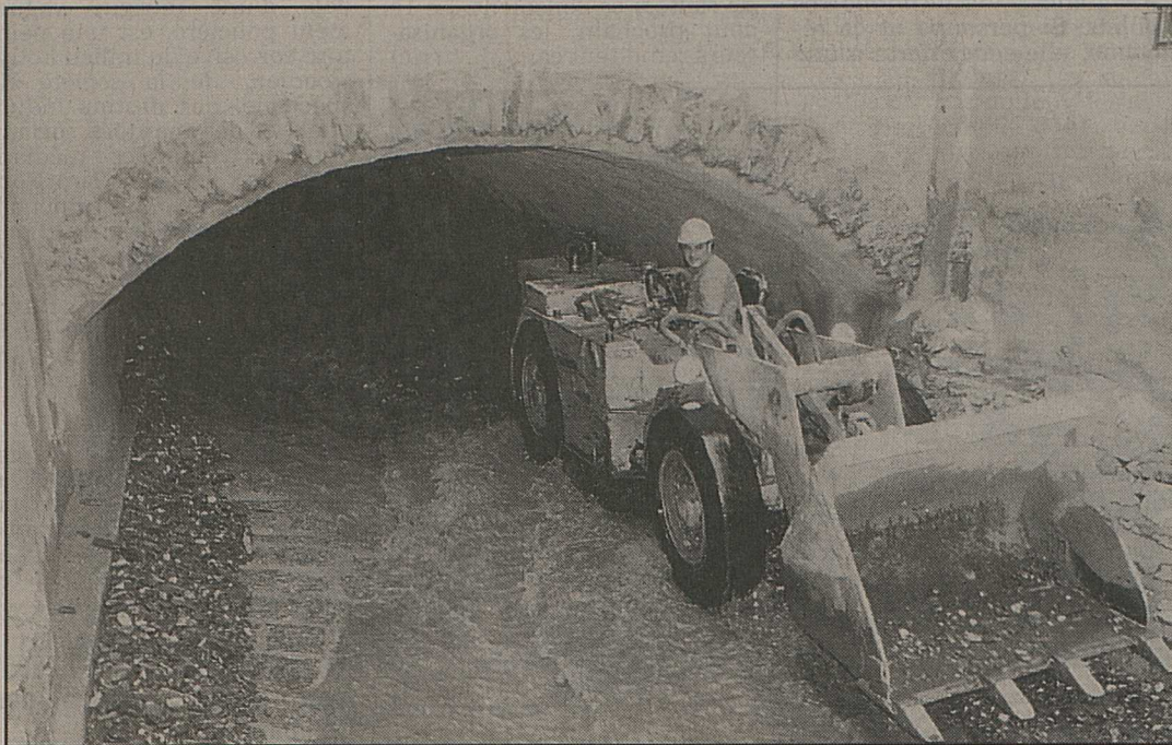
Une «marineuse», engin spécialement conçu pour travailler en galerie, a été engagé pour faire le ménage sous la rue du Rhône et la partie sud du Grand-Pont.
