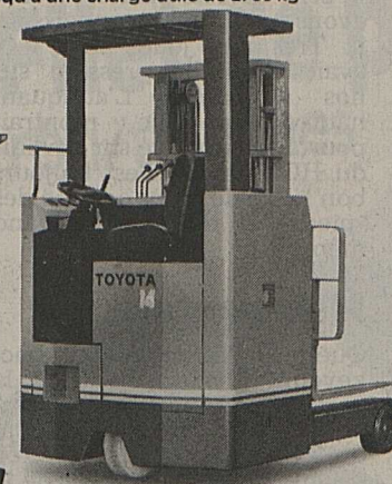
TOYOTA Chariot élévateur FBRE à mât retractable, jusqu'à une charge utile de 2750 kg
