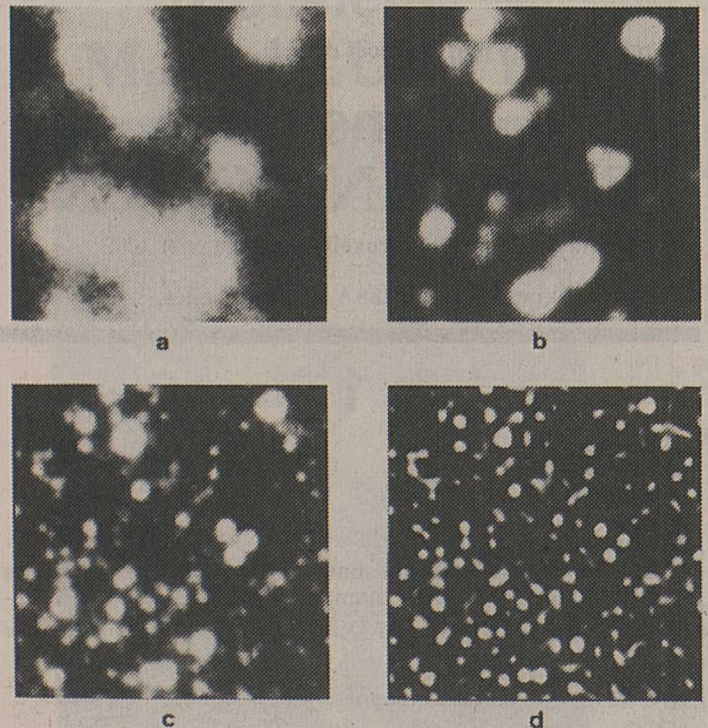
Les nouvelles techniques qu'utiliseront les deux télescopes fabriqués en Suisse permettent un gain considérable, illustré sur ces quatre images, selon que la nuit est agitée (a) ou calme (b): en haut, on distingue au mieux de dix à quinze objets célestes. Grâce aux nouvelles caméras électroniques (c), puis avec un traitement par ordinateur (d), on arrive à répertorier plus de cent objets astronomiques!
