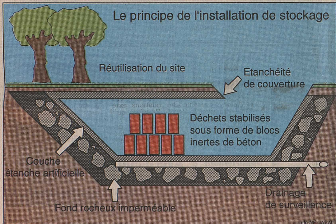
Un exemple théorique d'ISDS. Les critères les plus importants concernent la nature du fond rocheux, la qualité de la couche d'étanchéité et le contrôle des eaux de ruissellement et de drainage à la sortie de l'installation. Une structure surveillée.
