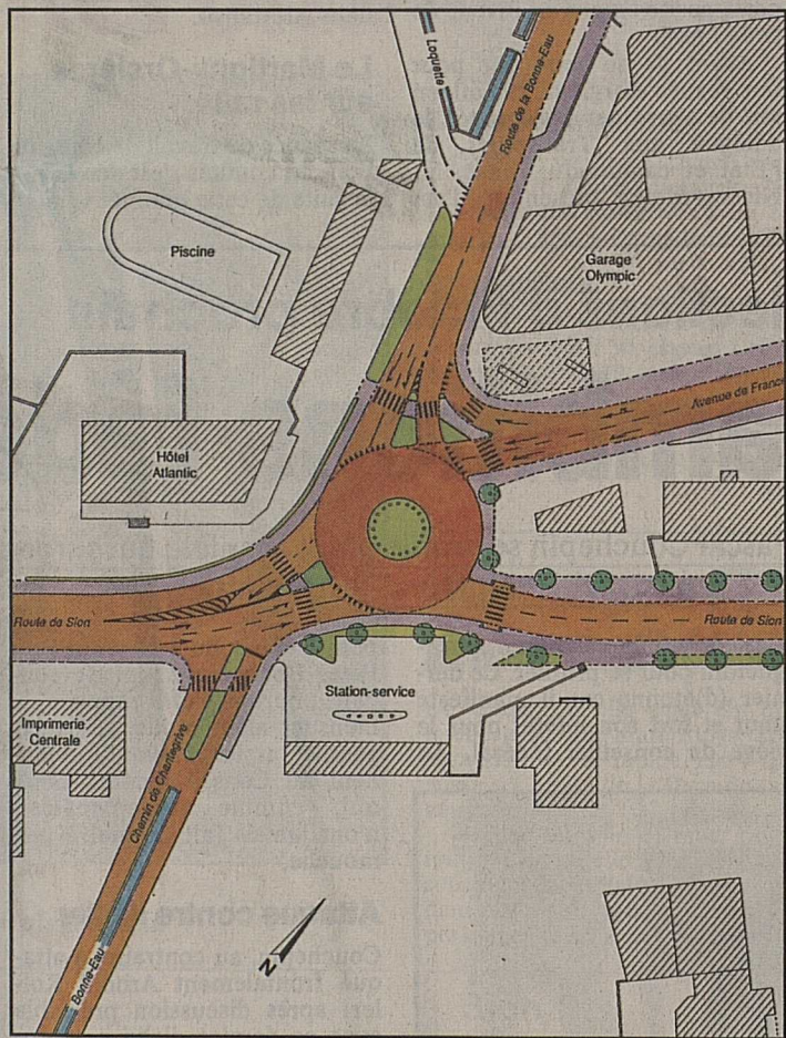
Le giratoire à cinq branches du carrefour Atlantic à l'entrée de Sierre. Les travaux débuteront cet automne. L'accès à l'hôpital de Sierre sera facilité.
