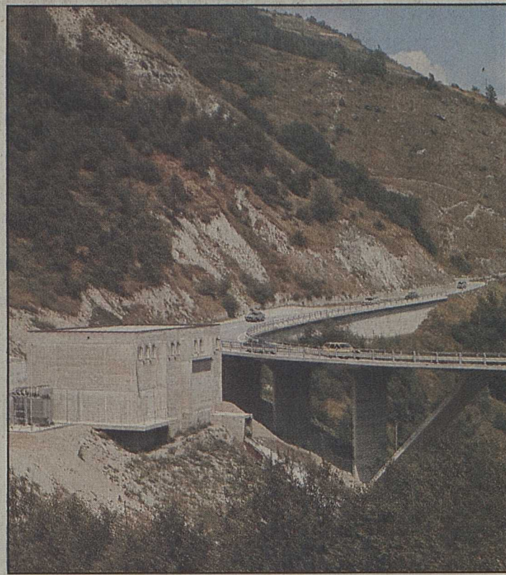
L'usine de l'aménagement de Leteygeon-Sauterot, en bordure de la route de Vex. La prise d'eau se trouve à proximité des pyramides d'Euseigne. Un exemple de solution régionale, solution d'avenir, solution écologique. Et c'est ce genre de solutions que l'initiative condamne à mort et que la loi pénalise grandement.
