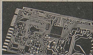
Ce circuit imprimé SMD développé par Miele commande tous les appareils Novotronic et il est à l'abri de toute usure.
