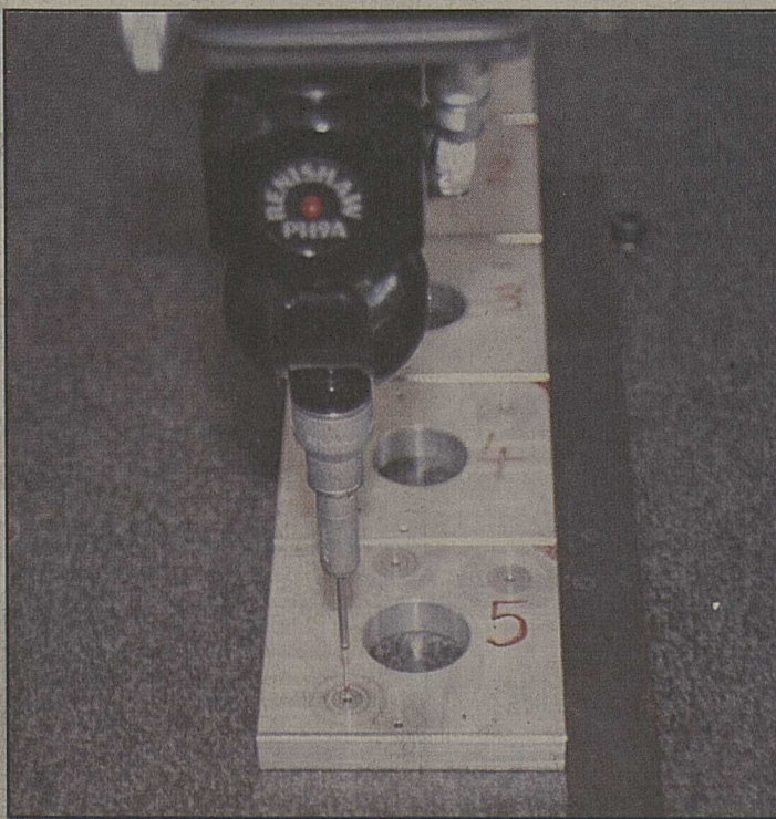
La tête au rubis mesure la pièce. Ses résultats seront comparés avec le profil introduit dans l'ordinateur.
