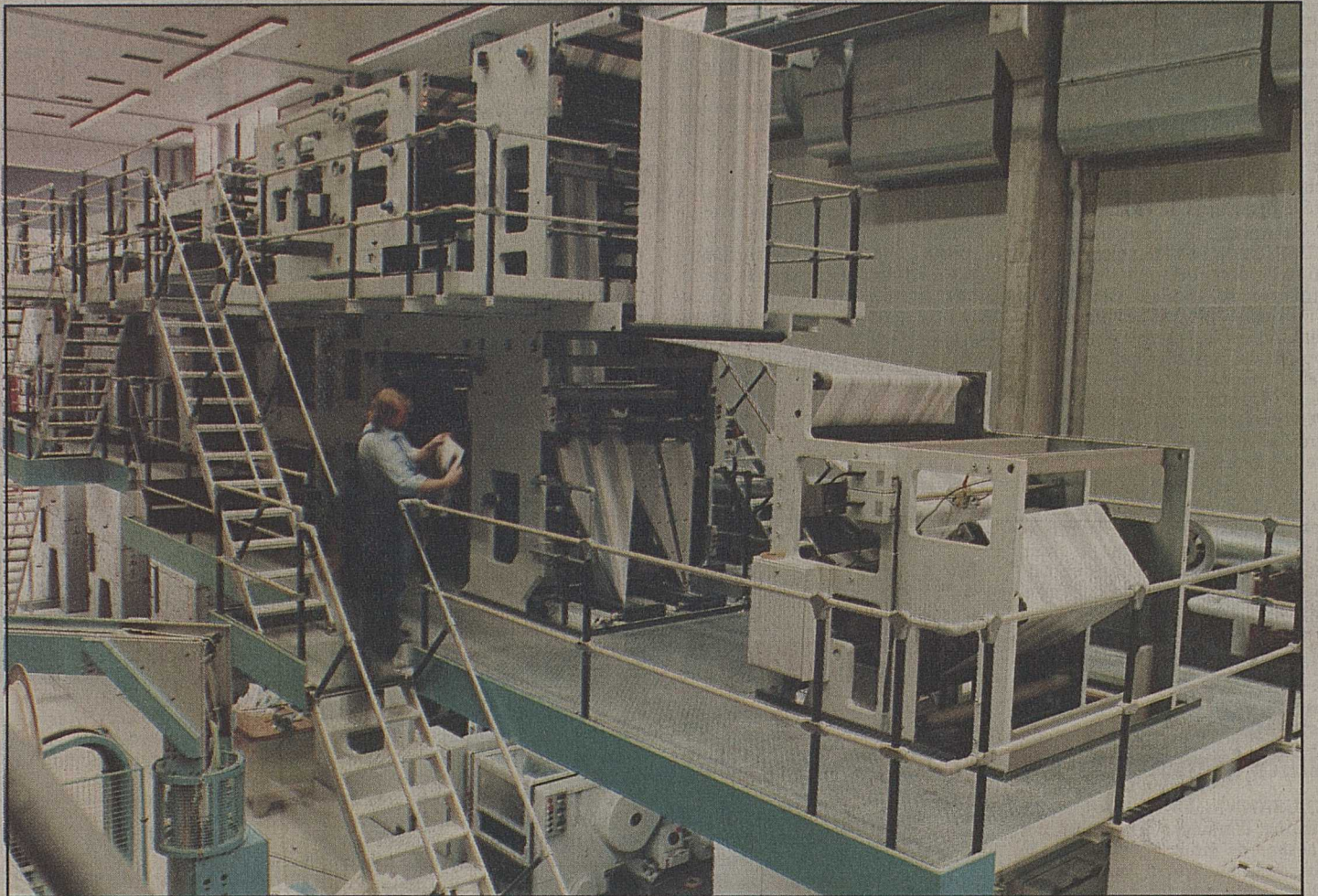
Vue partielle de la rotative Uniman installée au Centre d'impression des Ronquoz. C'est sur cette machine flambant neuve qu'a été tiré en grande première, cette nuit, notre quotidien.
