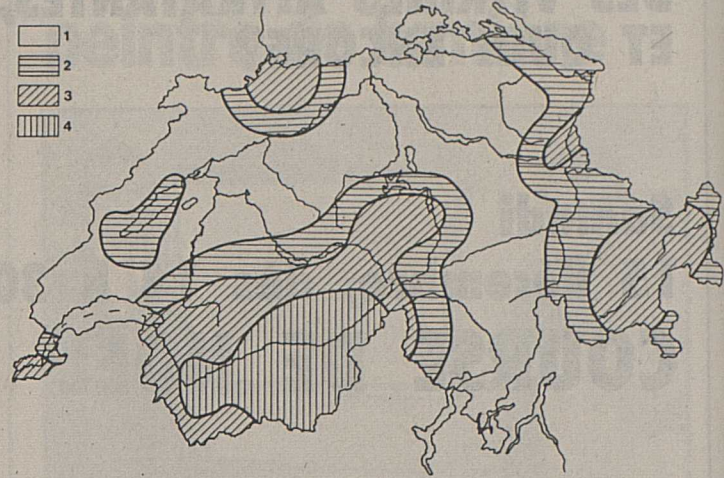
Carte du danger sismique en Suisse schématisée en quatre zones dans lesquelles règne un danger relativement 1. faible, 2. modéré, 3. moyen et 4. plus élevé. Carte éditée par les commissions suisses pour l'Unesco et la géophysique.
