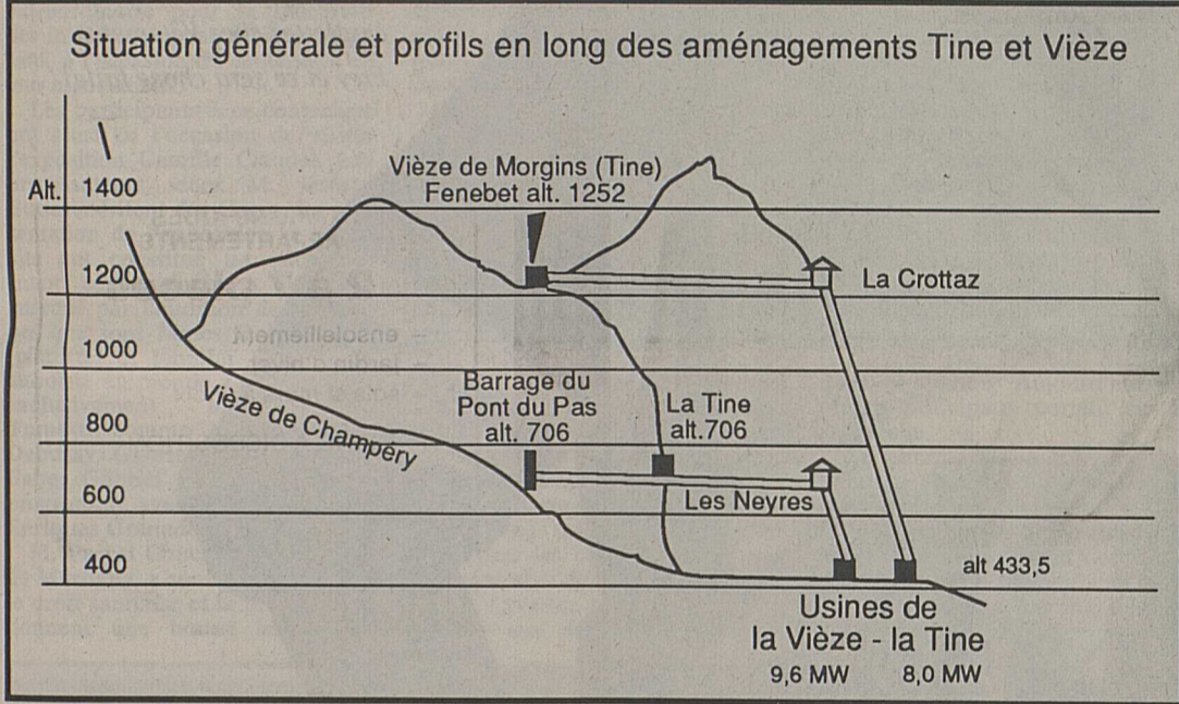
Profil en long des aménagements de la Vièze et de la Tine dont Ciba-Geigy est actuellement au bénéfice de concessions.
