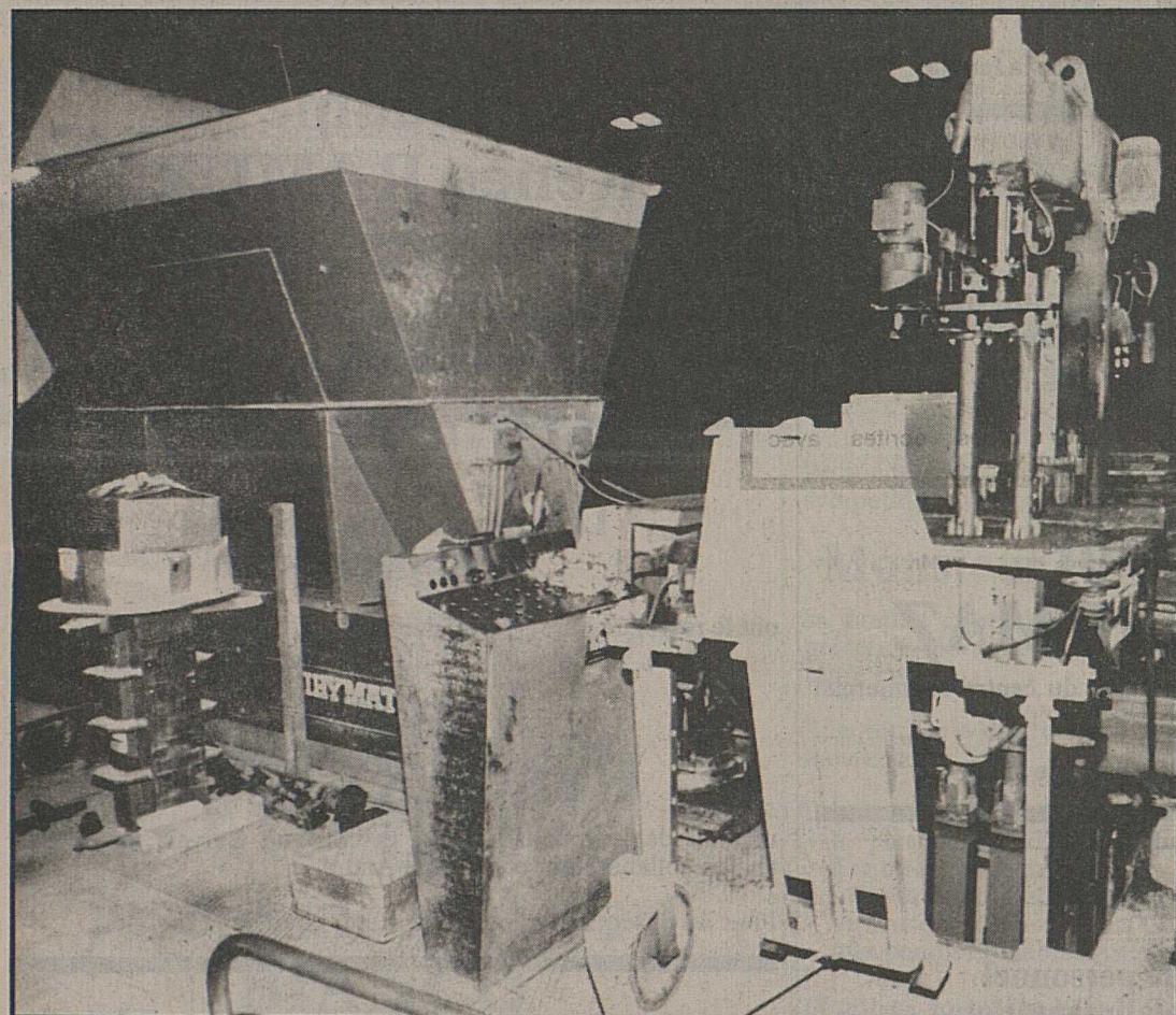
Machine à faire des tuyaux en béton d'un diamètre de 10 à 40 centimètres.
