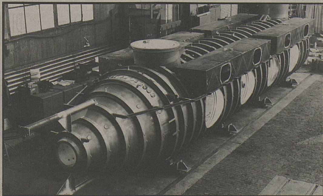
Le premier sous-marin panoramique suisse est actuellement en cours de construction chez Gebrüder Sulzer AG, à Winterthour.
