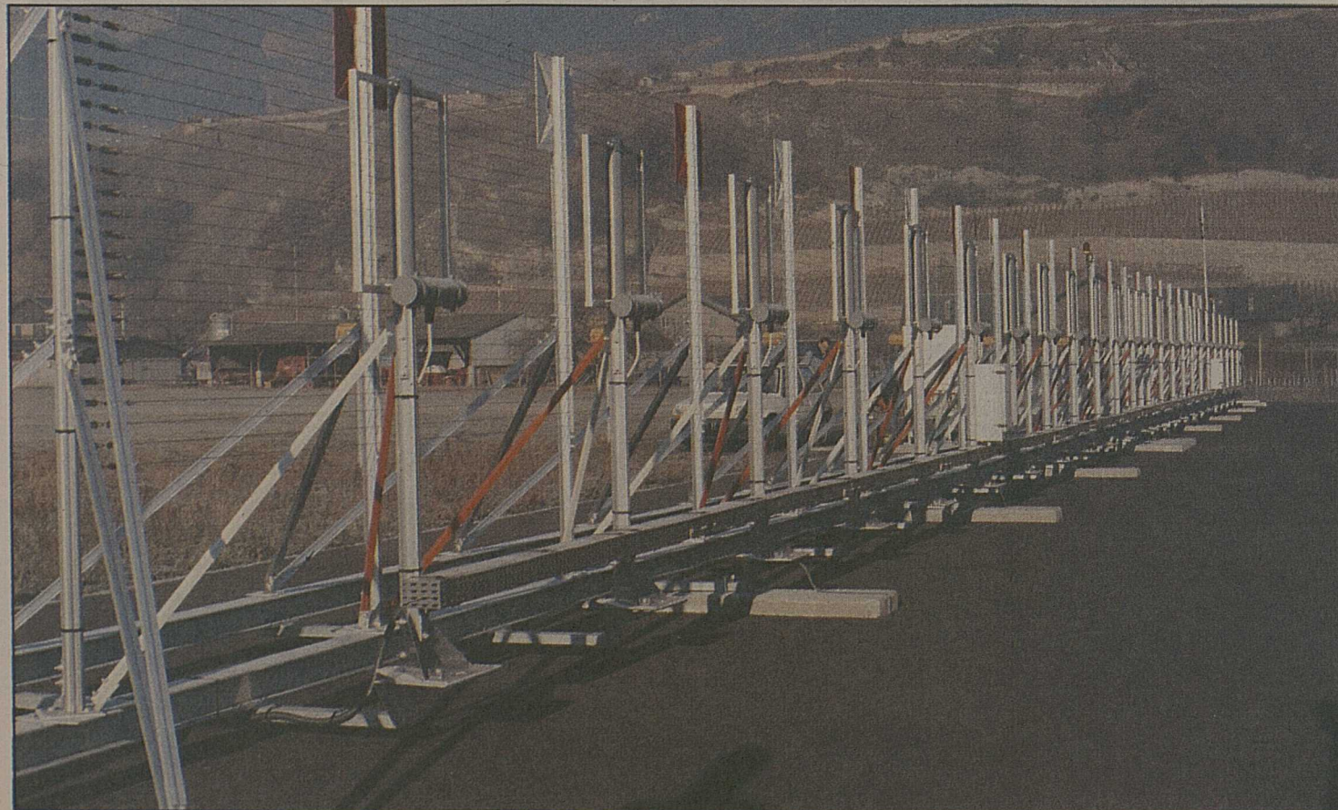
Le localizer, à l'extrémité ouest de la piste (côté Châteauneuf).
