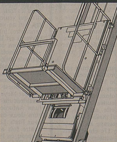
MAXIAL-SWISS "Universel" pour tous les métiers.
