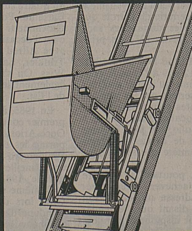
MAXIAL-SWISS "Spécial maçon" avec bac basculant automatique.
