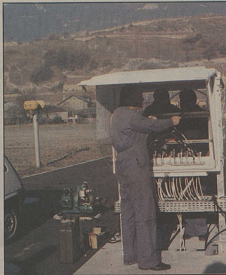
La mise en place par les spécialistes de Thomson-CSF et de Swisscontrol.
