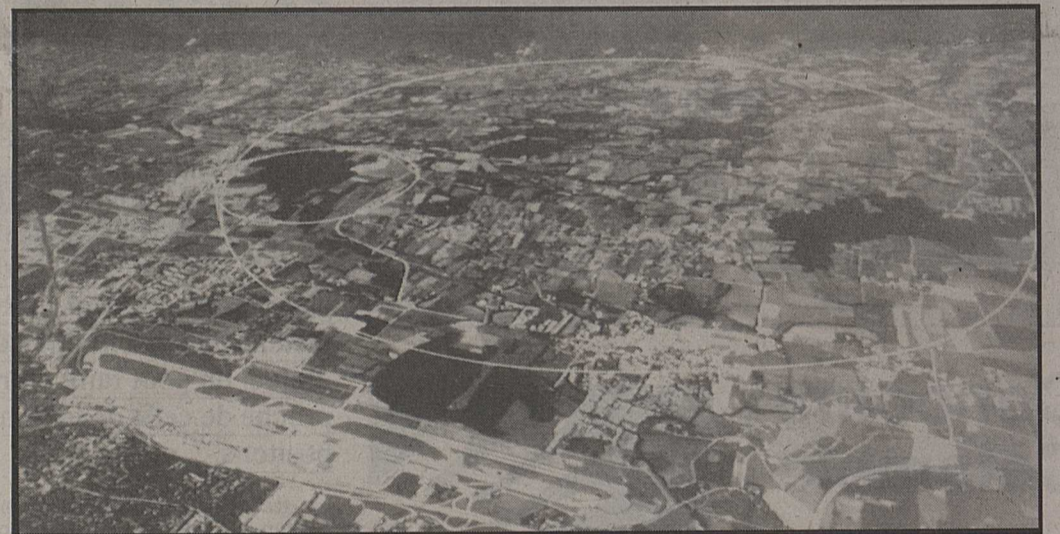
Sur cette vue aérienne, où l'on reconnaît au premier plan l'aéroport de Cointrin, on a dessiné le tracé du LEP. A l'intérieur de celui-ci, à gauche, on distingue le tracé de l'ancien accélérateur du CERN.
