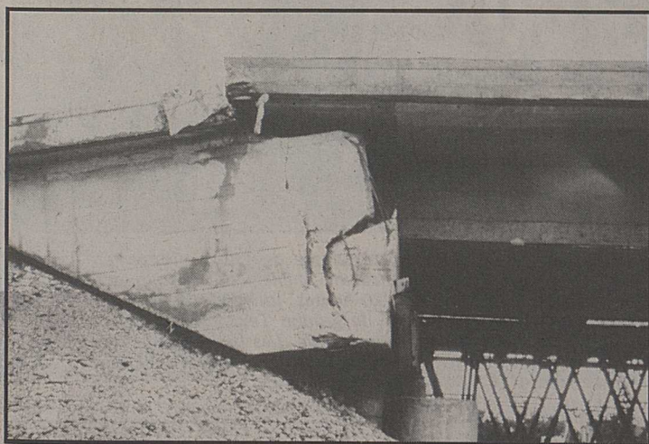
Pont détruit par l'effet bélier dans le Frioul en 1976.
