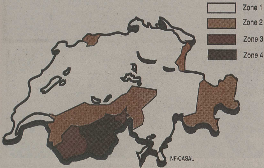
Sur cette carte établie par les sismologues à la demande des constructeurs de centrales nucléaires, on voit les quatre zones que compte notre pays. Les zones 3 et 4, les plus « dangereuses », couvrent globalement le Valais. En zone 2 se trouvent l'Oberland bernois, l'Engadine, l'est du canton de Saint-Gall et les alentours de Bâle. La zone 1, la plus « sûre », comprend l'essentiel du Plateau.
