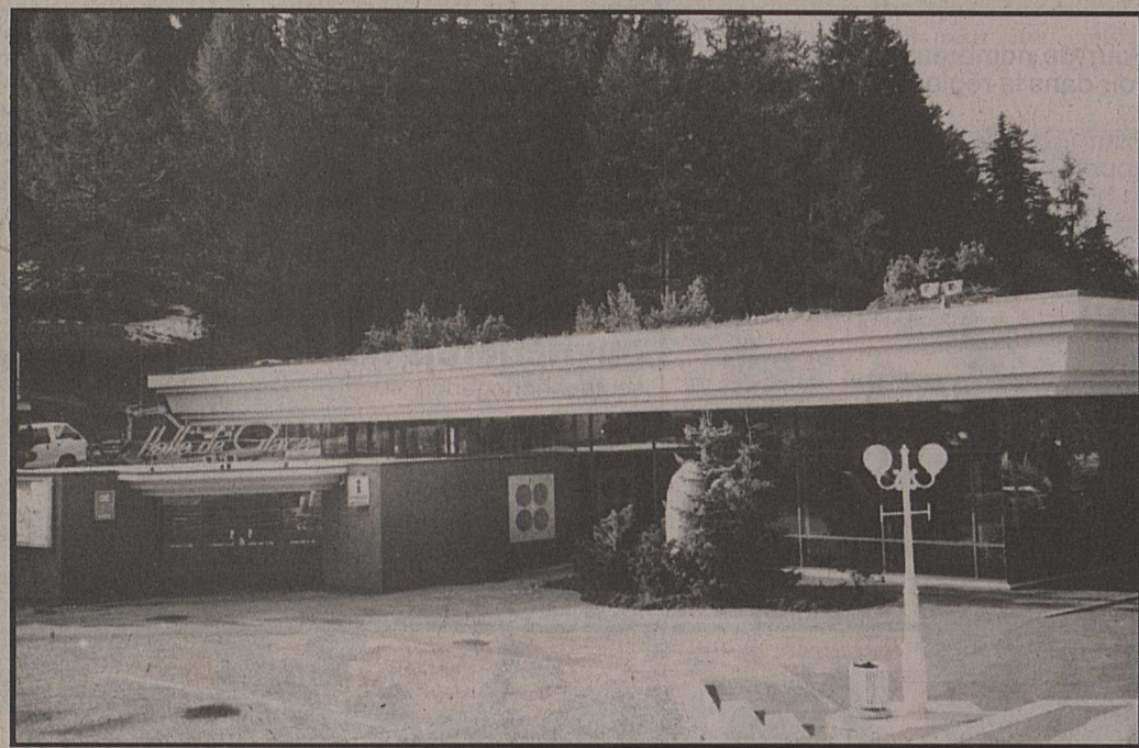
La halle de glace d'Y Coor. Depuis juin dernier, le fluage de la toiture ne s'est quasiment pas aggravé (2 mm de plus). Le toit du complexe risque en fait de se déformer l'hiver, poids de la neige oblige. Raison pour laquelle les travaux seront entrepris avant la morte saison.
