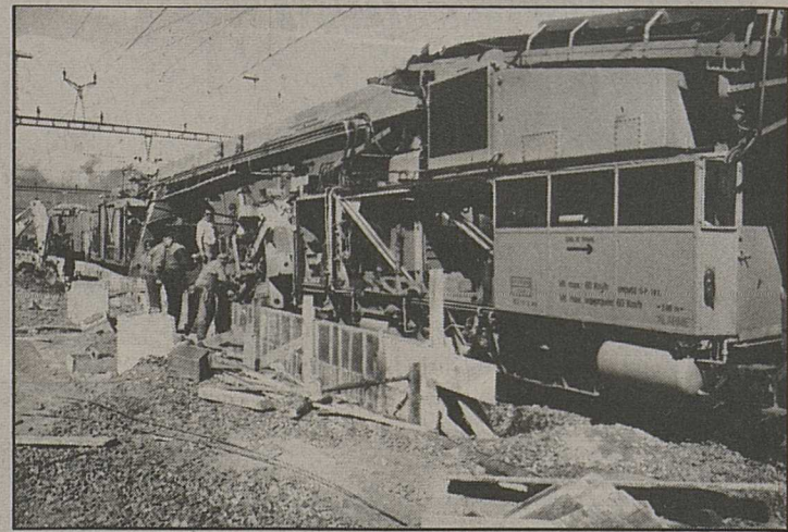
Utiliser des machines d'entreprises privées s'avère plus rationnel pour les CFF. Ici une DRL, «monstre» long de 220 m, qui crible le ballast avant de mettre en place les nouvelles traverses.
