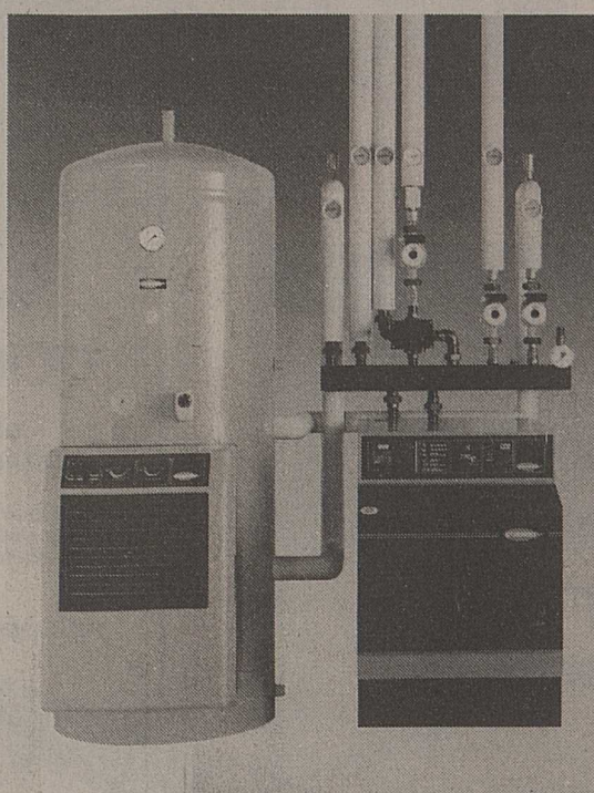
Centrale de chauffe avec ballon d'eau chaude et pompe à chaleur
