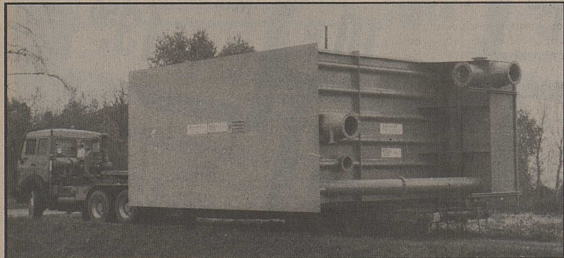
A la tombée du jour, mardi dernier, le convoi transportant ce filtre de 15 tonnes est prêt à prendre la direction de la RN 9 à partir de Collombey-le-Grand.
