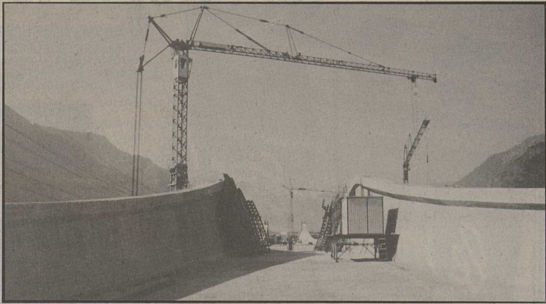
Le nouveau pont de Riddes. Les deux rives se sont serré la main jeudi à 2 heures du matin.
