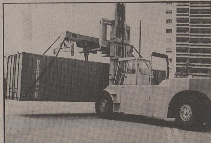
A l'heure du chargement des containers sur le train. Cet élévateur géant peut soulever la bagatelle de trente tonnes.
