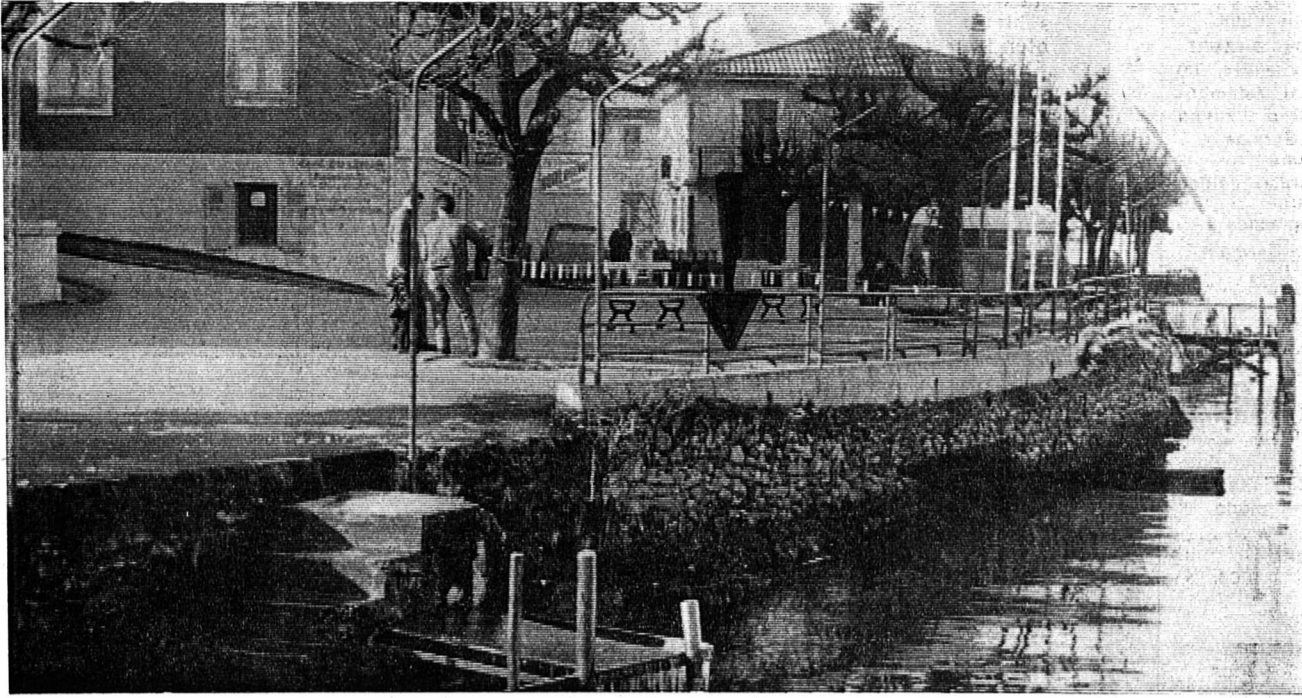
Une vue partielle du quai avec (flèche verticale) l'endroit où le quai est fissuré sur une dizaine de mètres avec une largeur de fissure variant entre 5 et 10 cm. Les « gallions » (flèche horizontale) ont été poussés par les vagues sous-lacustres, à leur base, perdant ainsi une assise qu'on leur avait donnée.
