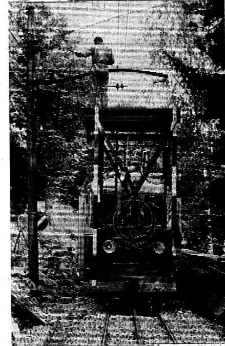
La journée, une équipe de spécialistes de l'AOMC procède au réglage de la ligne aérienne. Il s'agit pour elle de relever toute la ligne de 20 à 30 cm suivant les endroits.
