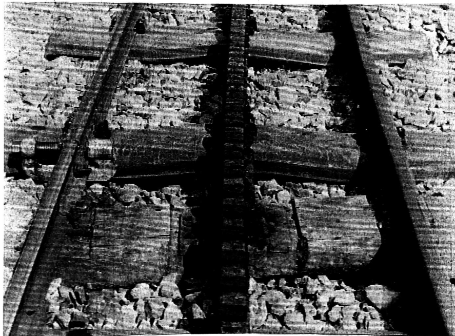
A la jonction de l'ancienne et de la nouvelle voie on distingue nettement au premier plan les anciennes traverses en bois, et au second plan les nouvelles en fer avec le dos d'âne permettant le fixage de la crémaillère.
