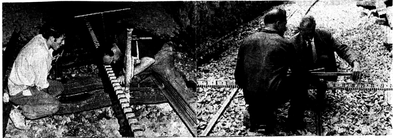
Tandis qu'une équipe pose traverses et voies neuves, une autre est occupée à la pose des écrous et au réglage préliminaire de la voie. ★ Le directeur Kuhn, aidé d'un chef d'équipe, procède au réglage de la voie qui exige beaucoup d'attention.
