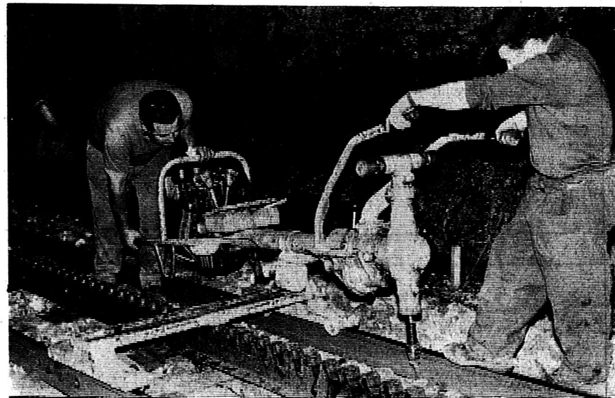
Pour déboulonner les voies tenues aux traverses par des écrous, une machine spéciale est utilisée, accomplissant ce travail avec diligence. Le même procédé est utilisé pour la fixation des traverses de fer aux nouvelles voies, par les écrous (dans le cercle).
