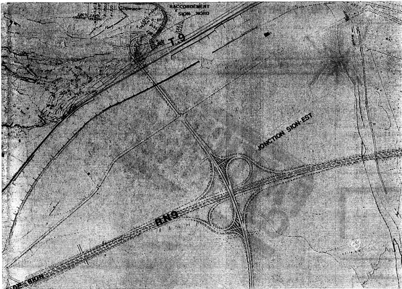
Les plans de la route de transit sud avec le raccordement Sion Nord (trait renforcé). Au sud, le tracé de la route nationale 9 (future autoroute), avec la bretelle de sortie et d'entrée. Début des travaux en 1972.
